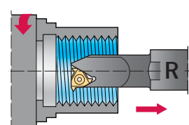
Левая резьба правая державка правая пластина обратный угол наклона
